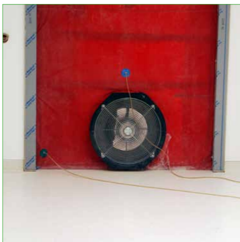
Blowerdoortest
